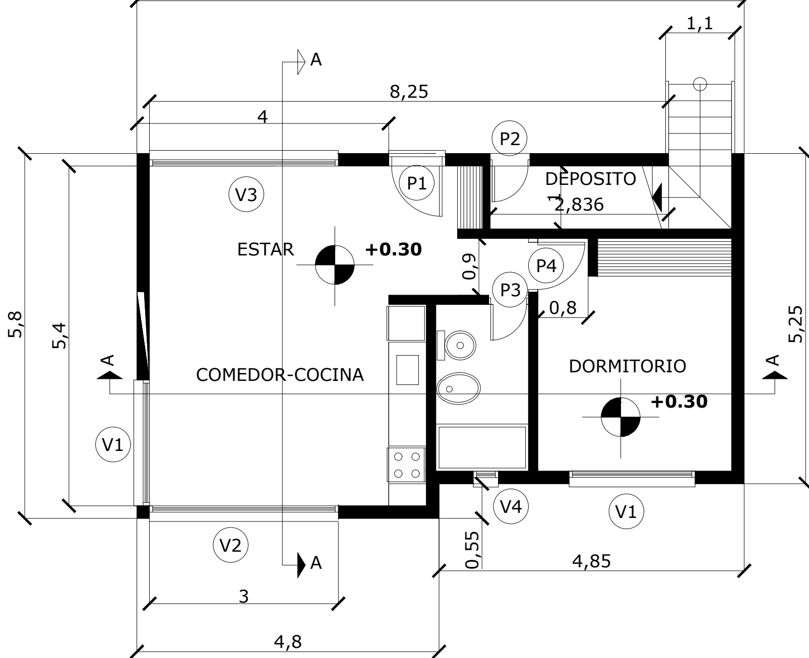
PLANTA BAJA
